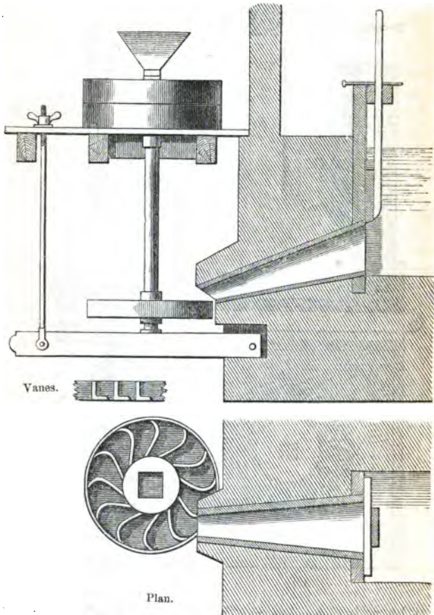
Fig. 9.—Rouet Volant.
